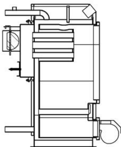
Fig 1. Funcționarea cazanului
