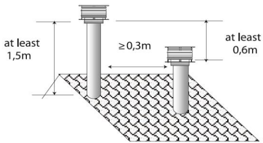
Fig 3. Distanța între coșurile de fum
